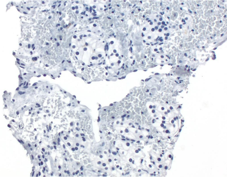
TIROGLOBULINA, 20X
