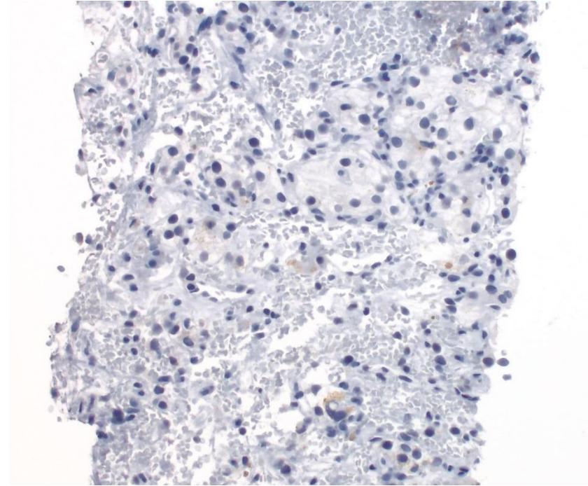
TTF1, 20X
